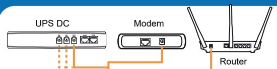
Modem y Router con igual voltaje de alimentación
